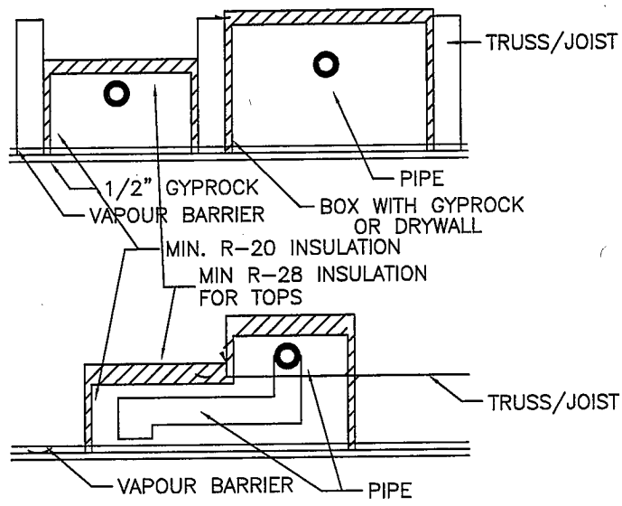
INSULATION DETAIL N.T.S.
